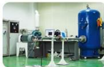
유동저항 시험기(컨버터)
